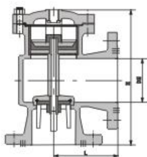
H142X 结构图
