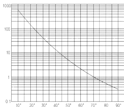
流量曲线图
