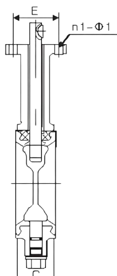
KDA71/371X10 KDA71/371-16 结构图
