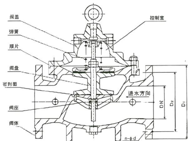
800X 结构图
