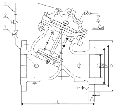
1.过滤器 2.针阀 3.小球阀
