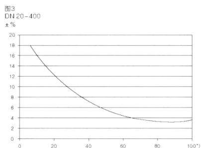
KFSPX 流量图
