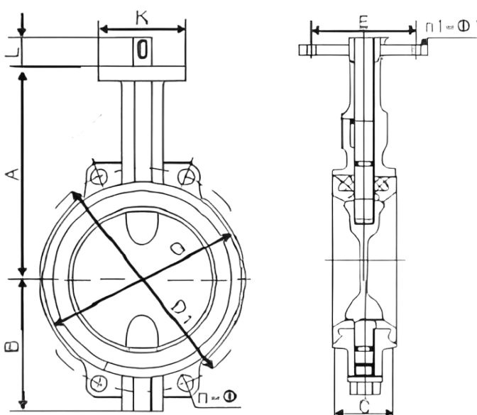
KD71/371X-10/16 结构图
