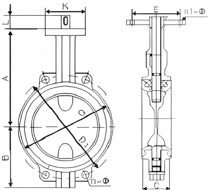
KD71、3/6/971X-10 KD71、3/6/971X-16 结构图
