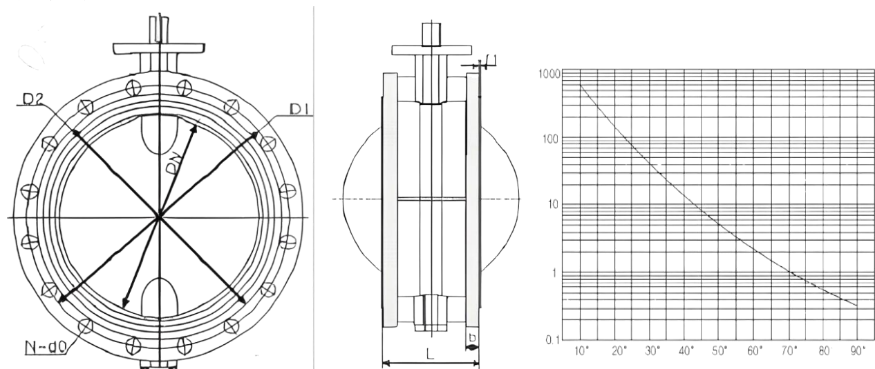
KD41、3/6/941-10 KD41、3/6/941-16 结构图
