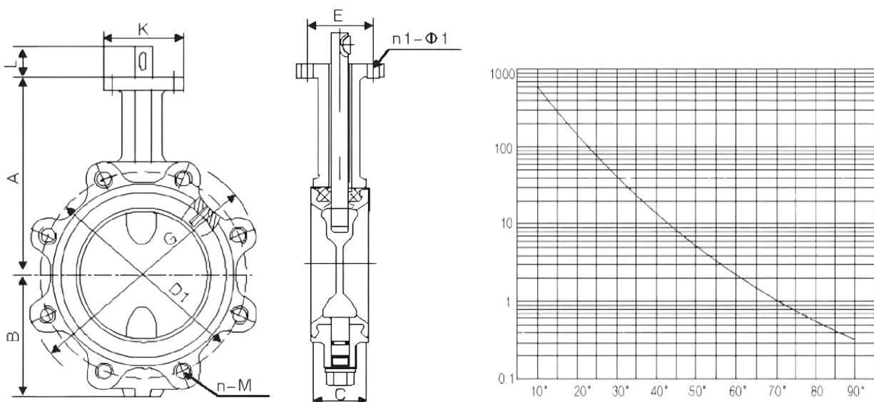
KDA71、3/6/971X-10 KDA71、3/6/971X-16 结构图
